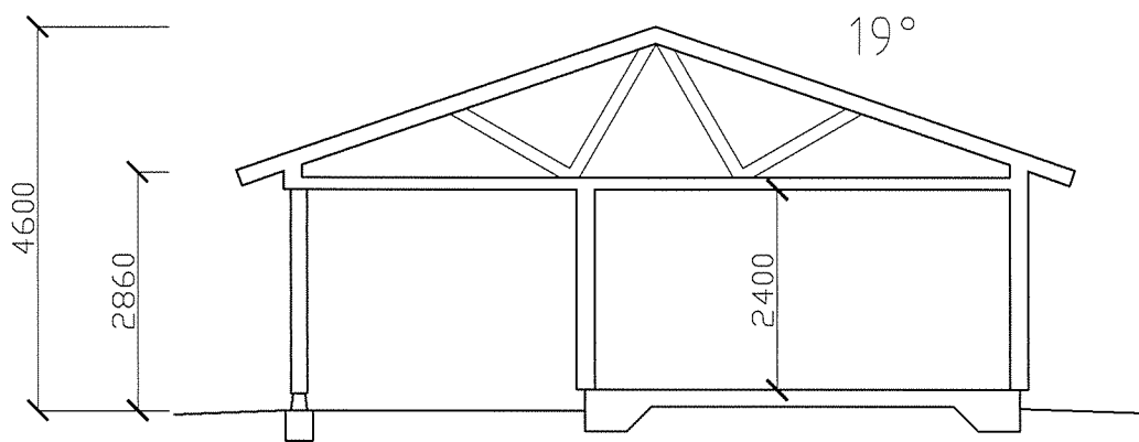
SEKTION A-A
