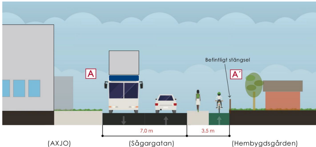
Sektionsbild för möjlig utformning på Sägargatan (Se föregående bild A - A' .)
