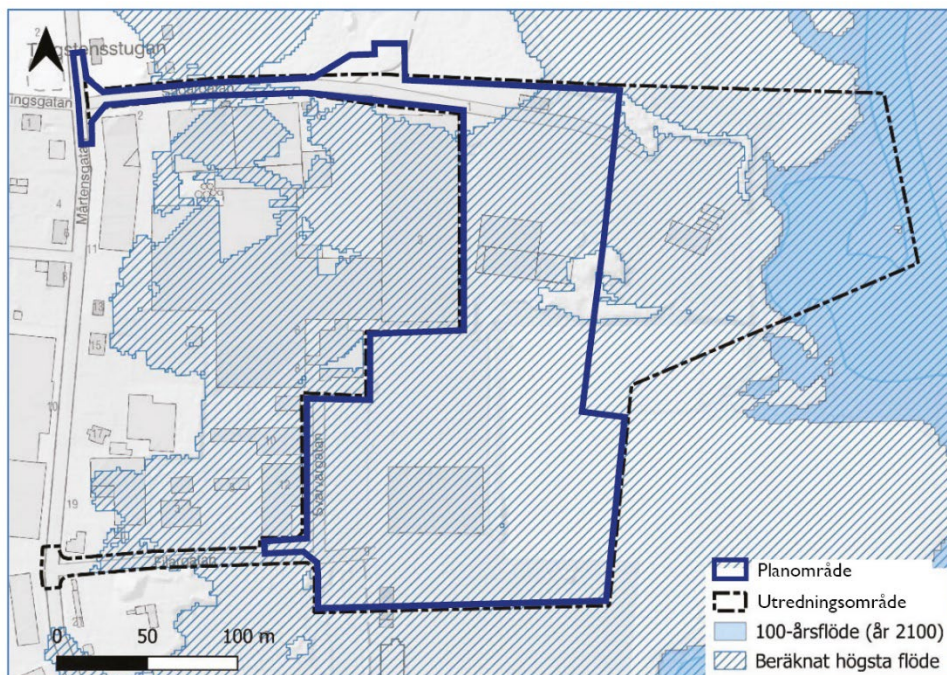
Översvämmande ytor vid 100-års flöde och vid beräknat högsta flöde. Källa: MSB 2025
